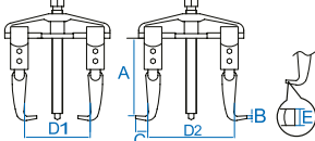
Äußeres Abziehen
