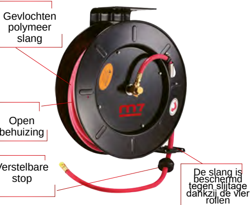
SA4_A PNEUMATISCHE SLAGHASPEL
